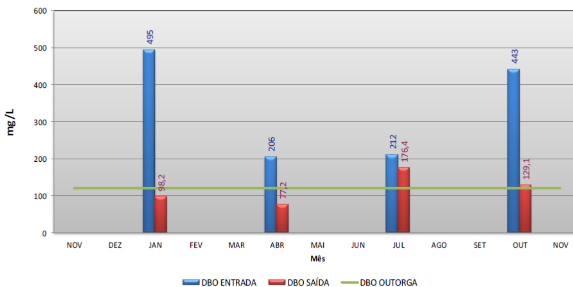
Figura AC-183 - Resultados de DBO da ETE Pacotuba.
