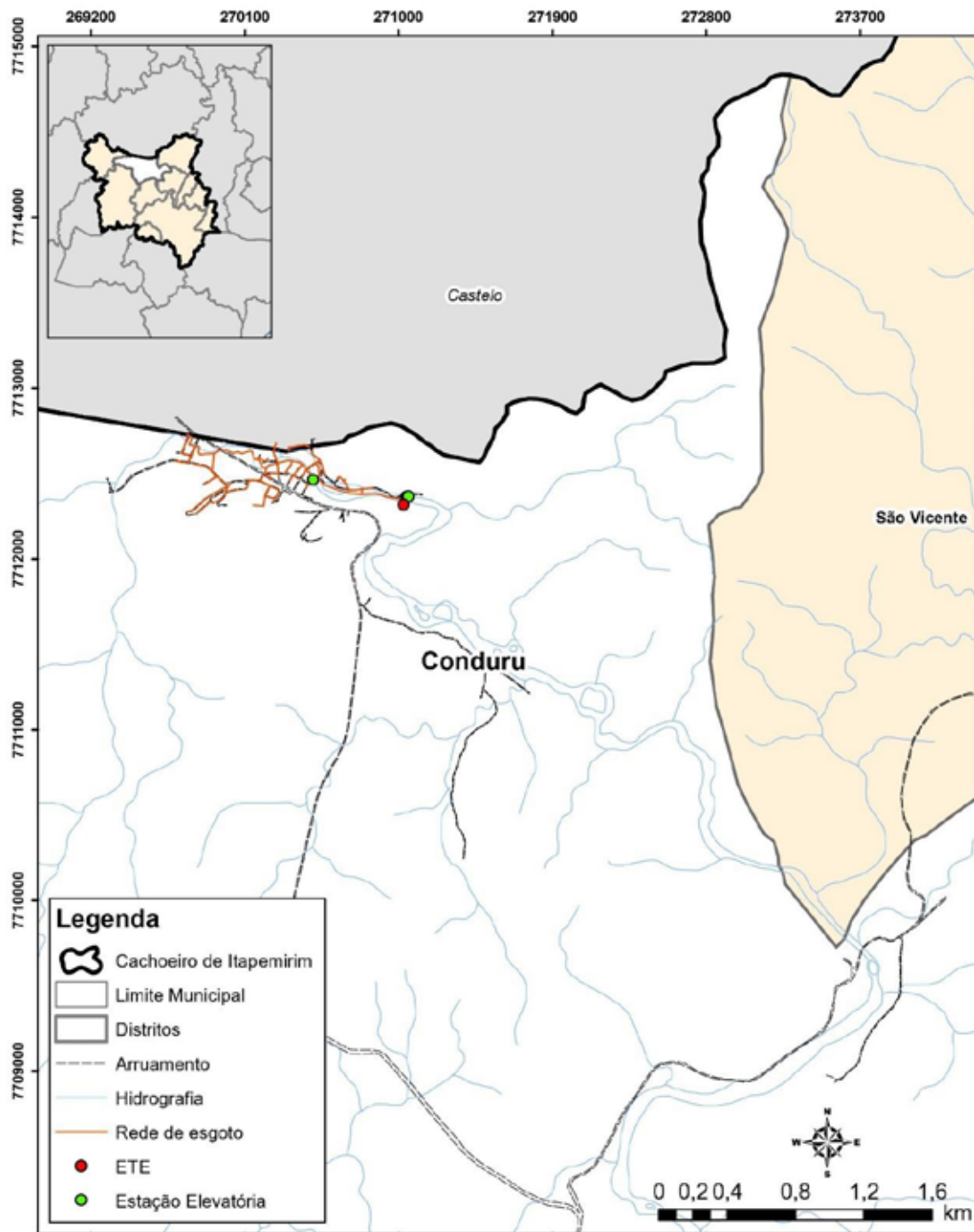
Figura D-198 - Sistema de esgotamento sanitário do distrito Conduru.
