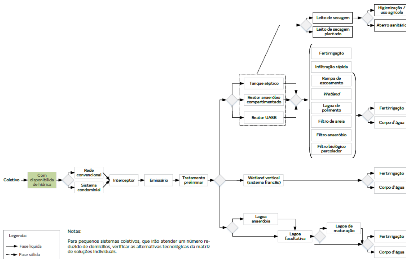
Figura O-285 – Matriz tecnológica de soluções coletivas para o esgotamento sanitário.
