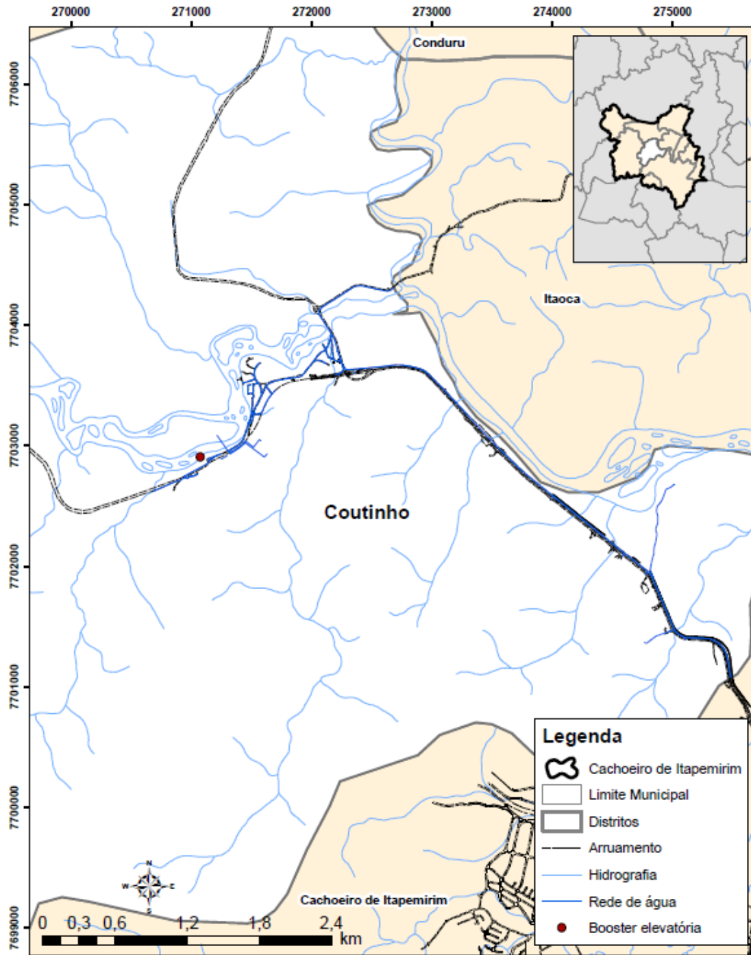
Figura C-189 - Sistema de abastecimento de água do distrito de Coutinho.
