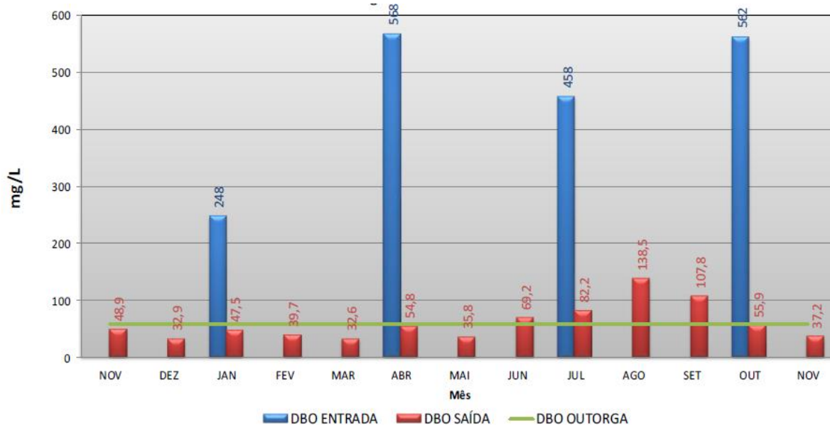
Figura AC-176 - Resultados de DBO na ETE Alto Moledo.
