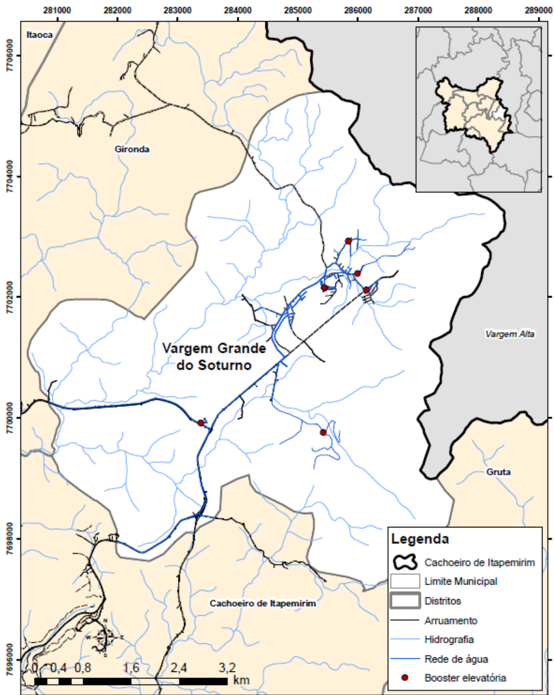
Figura C-193 - Sistema de abastecimento de água do distrito de Vargem Grande do Soturno.
