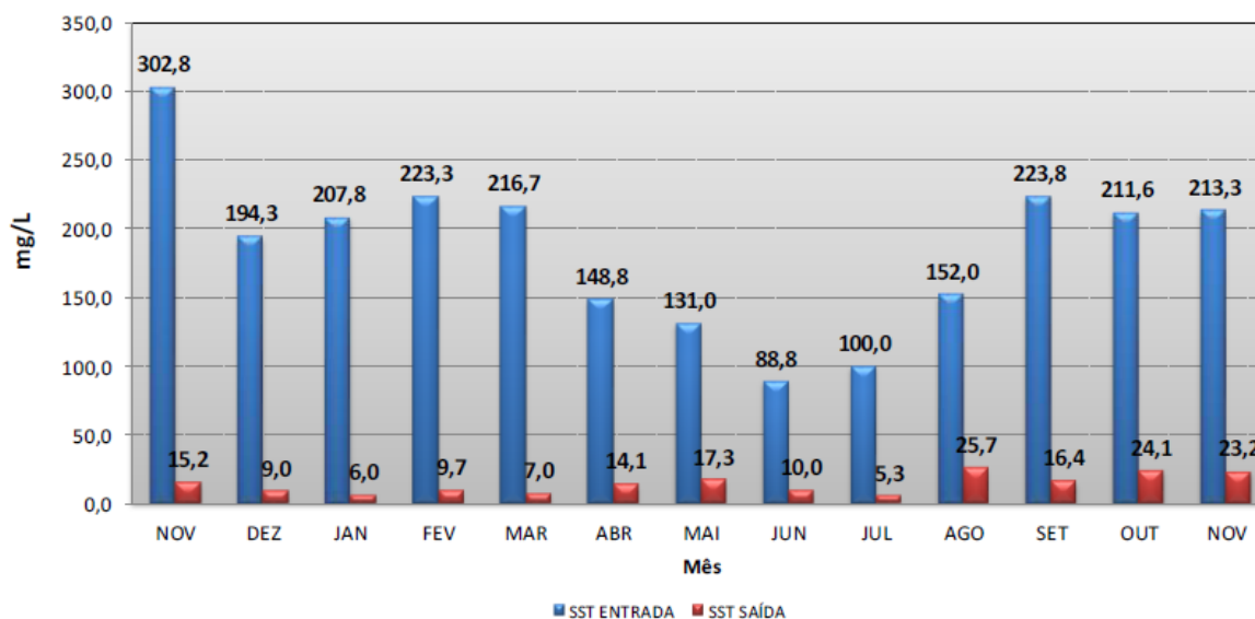
Figura AC-175 - Valores médios de SST da ETE Coronel Borges.
