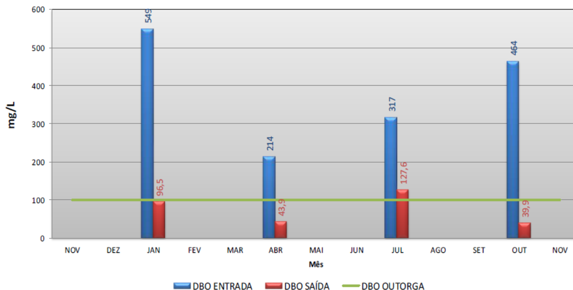
Figura AC-180 - Resultados de DBO na ETE Coutinho.
