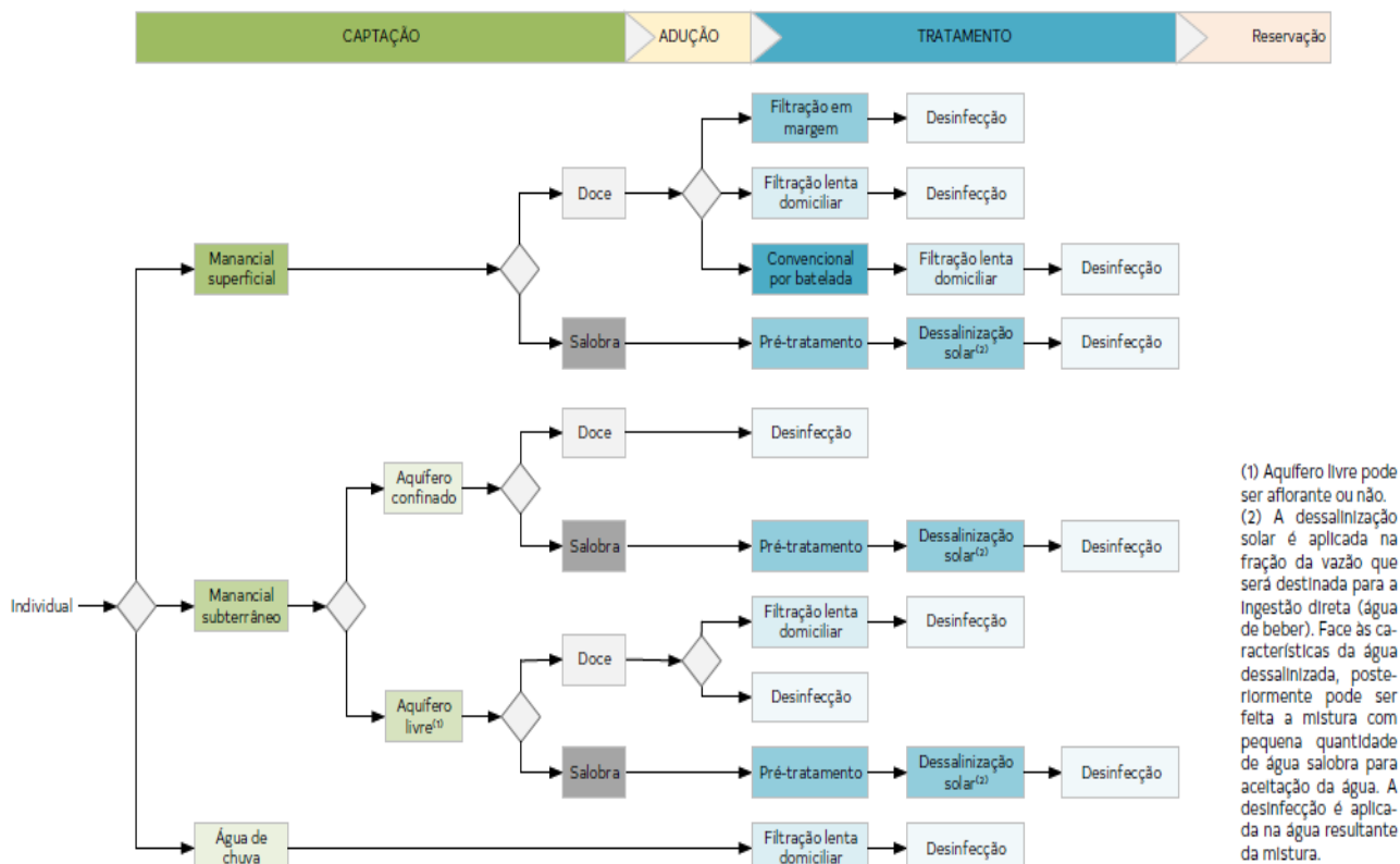
Figura O-284 – Matriz tecnológica de soluções individuais para o abastecimento de água.
