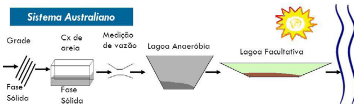
Figura 16-161 - Etapas de tratamento de esgotos pelo sistema australiano.
