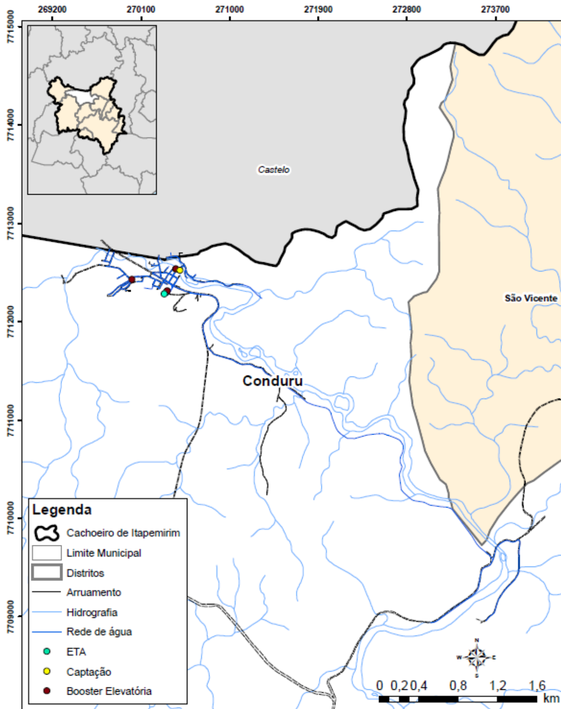
Figura C-187 - Sistema de abastecimento de água do distrito de Conduru.
