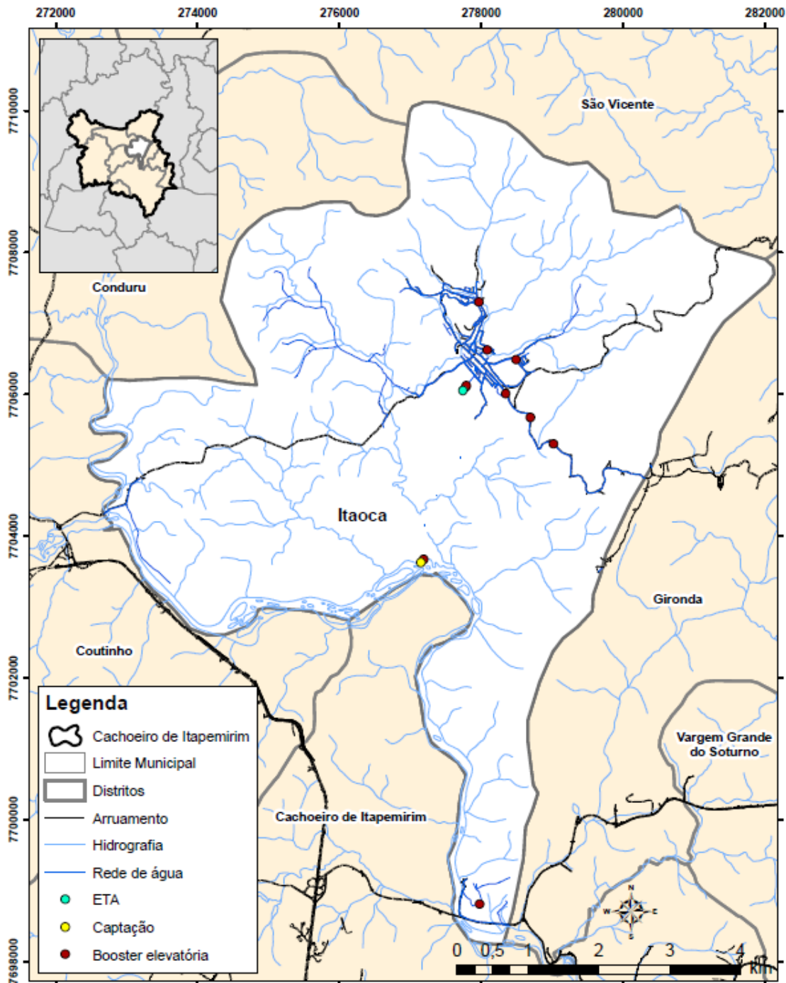
Figura C-191 - Sistema de abastecimento de água do distrito de Itaoca.
