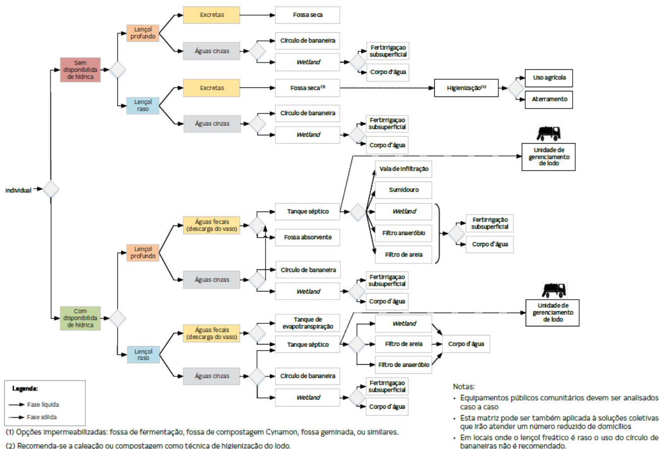
Figura O-286 – Matriz tecnológica de soluções individuais para o esgotamento sanitário.
