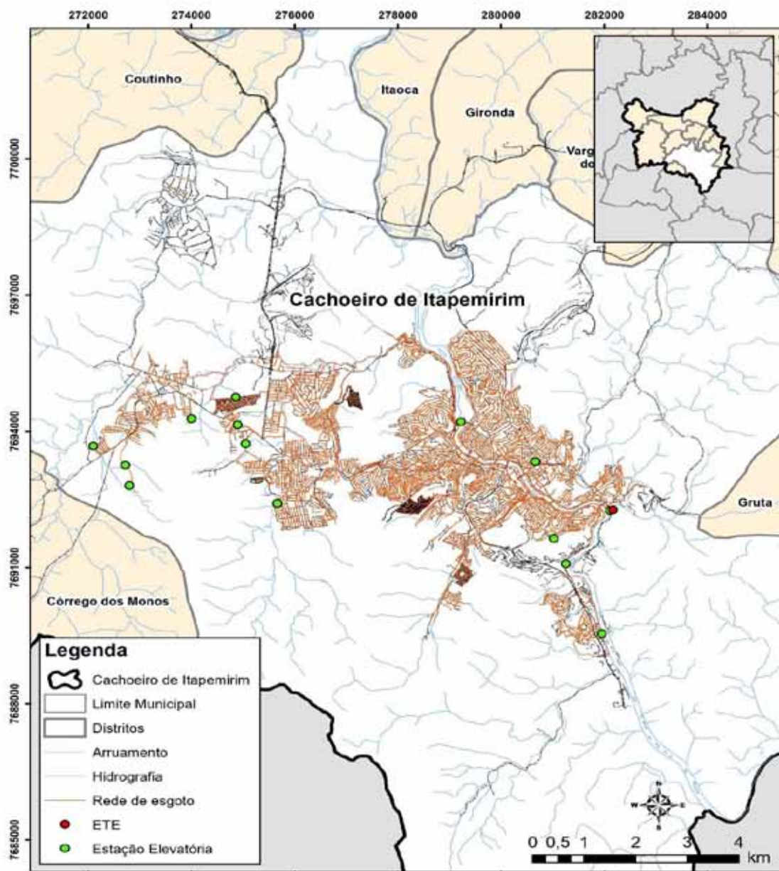
Figura D-196 – Sistema de esgotamento sanitário da Sede Municipal.
