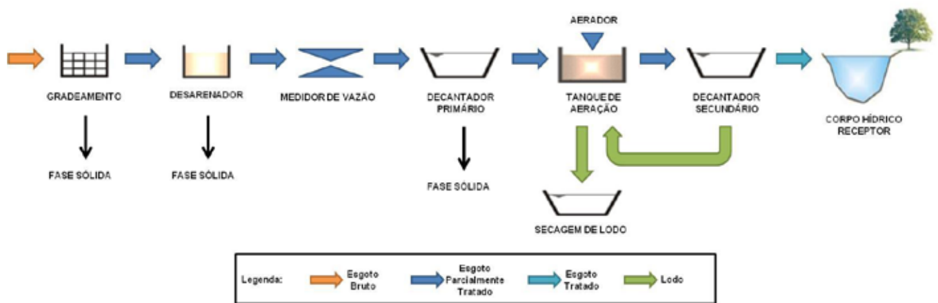
Figura 16-163 - Etapas de tratamento de esgotos pelo sistema de lodos ativados convencional.
