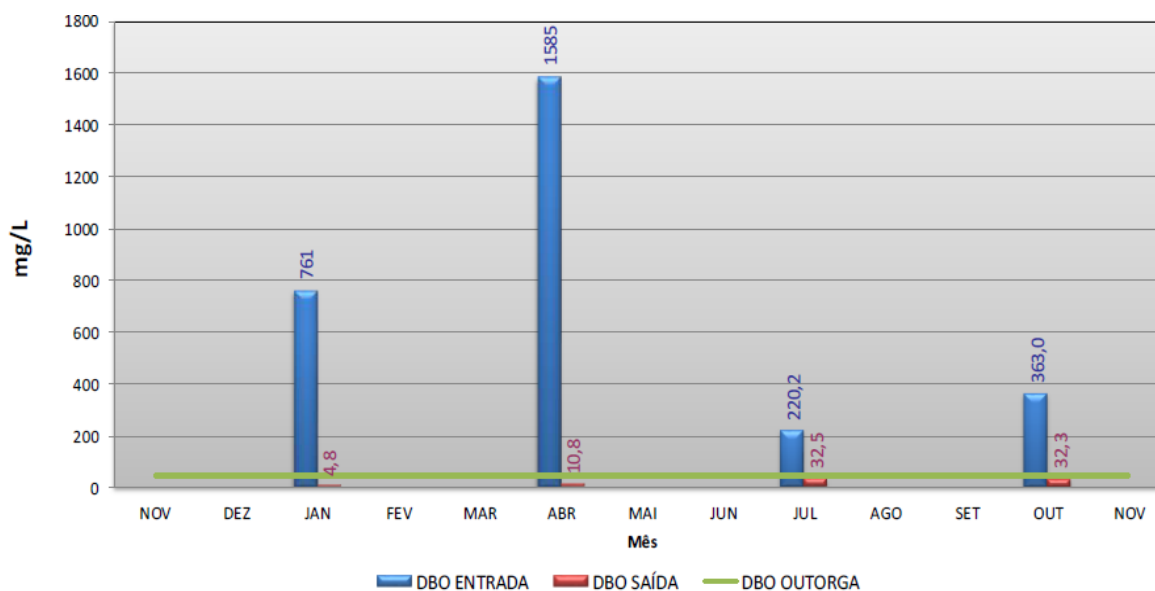
Figura AC-185 - Resultados de DBO da ETE Soturno.
