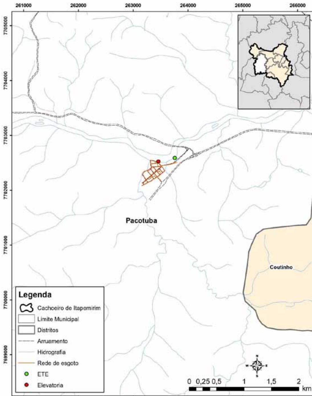
Figura D-203 - Sistema de esgotamento sanitário do distrito Pacotuba.
