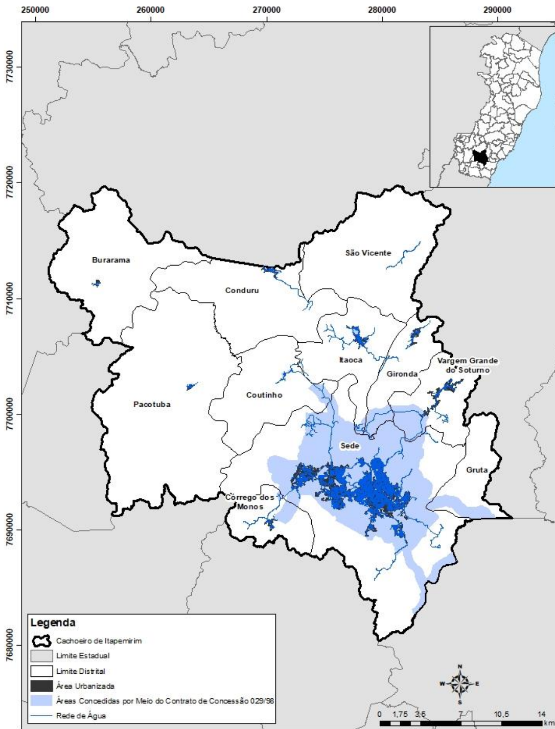
Figura O-248 - Áreas concedidas à BRK para abastecimento de água em Cachoeiro de Itapemirim pelo Contrato n.º 029/928, com destaque à atual rede de distribuição.
