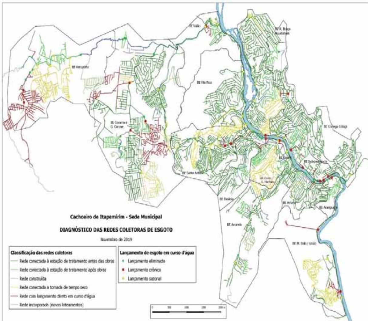
Figura 10-124 – Mapa das redes coletoras de esgoto da sede municipal após Projeto Tratar.
