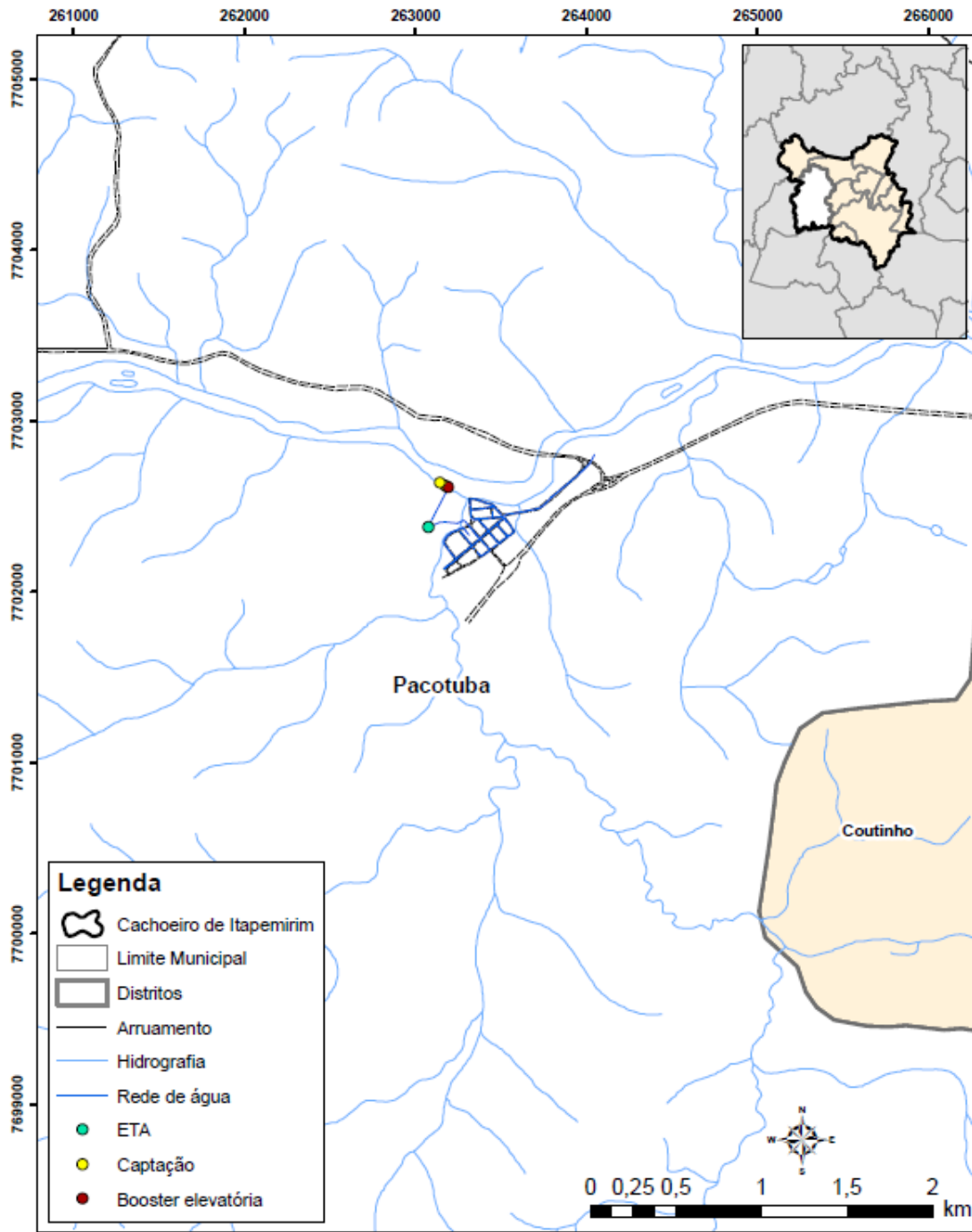
Figura C-192 - Sistema de abastecimento de água do distrito de Pacotuba.
