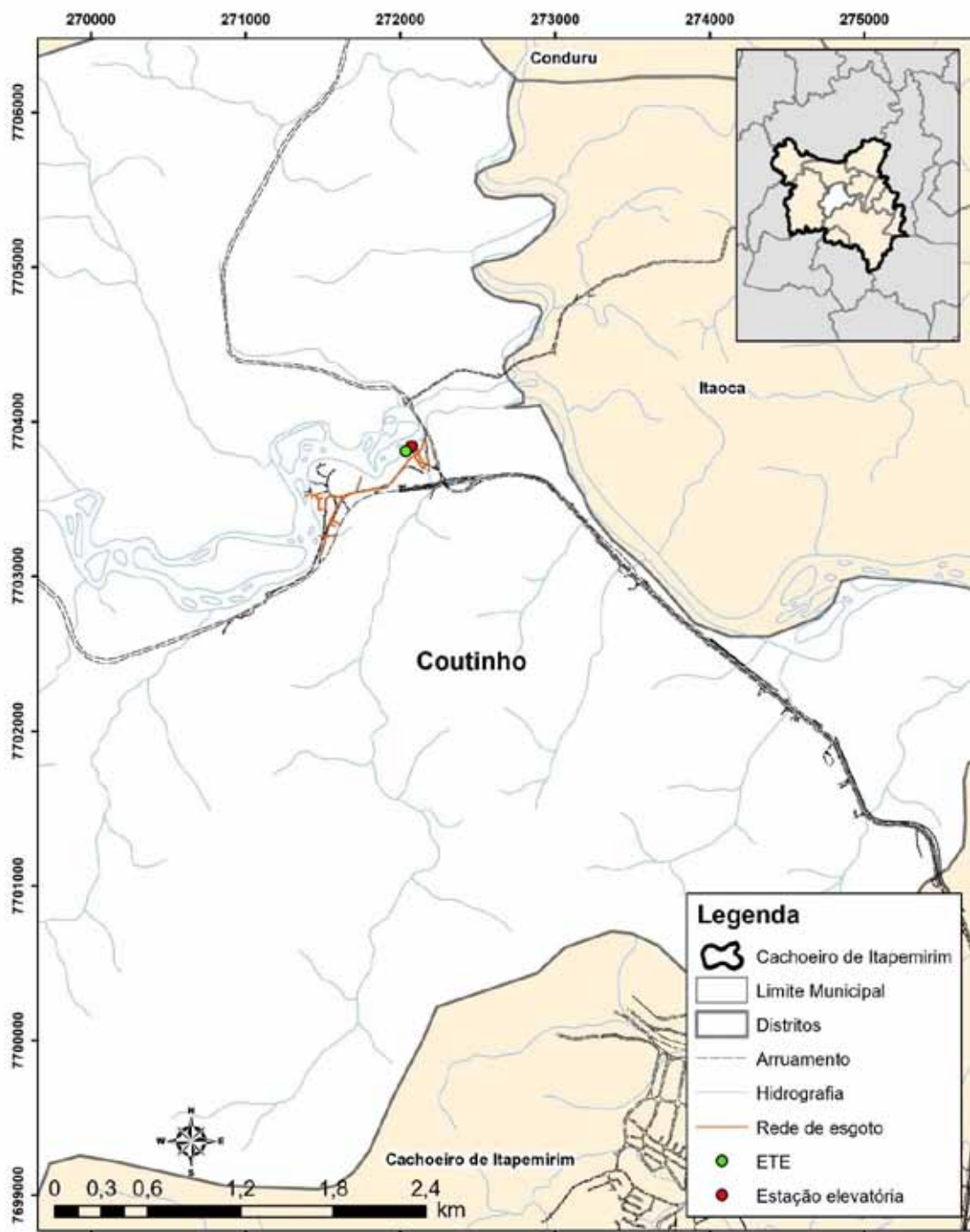
Figura D-200 - Sistema de esgotamento sanitário do distrito Coutinho.
