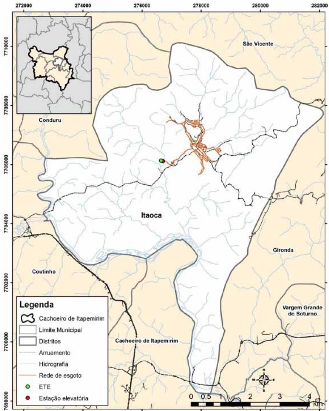
Figura D-202 - Sistema de esgotamento sanitário do distrito Itaoca.
