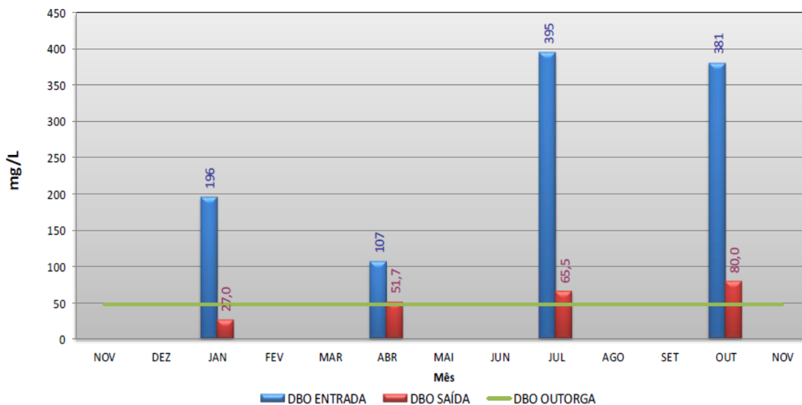
Figura AC-177 - Resultados de DBO da ETE Burarama.
