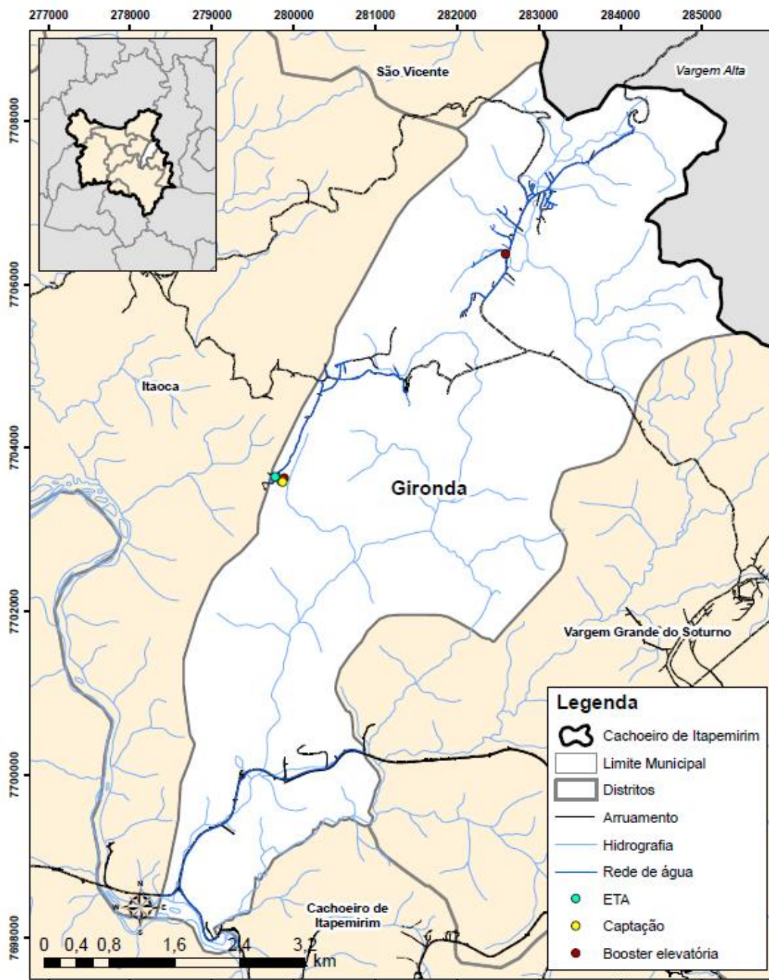
Figura C-190 - Sistema de abastecimento de água do distrito de Gironda.
