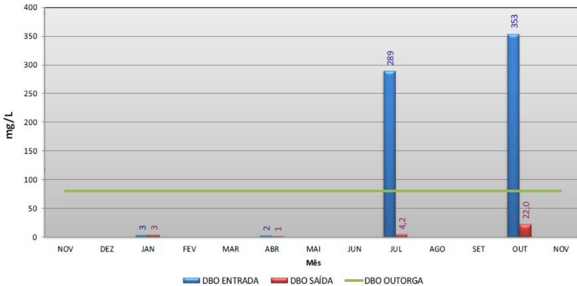
Figura AC-184 - Resultados de DBO da ETE São Vicente.
