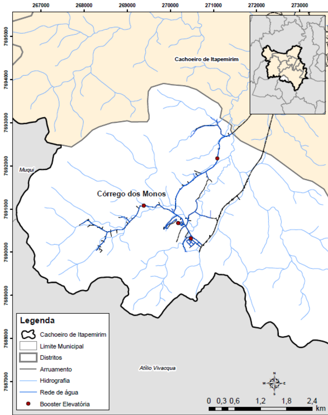
Figura C-188 - Sistema de abastecimento de água do distrito de Córrego dos Monos.
