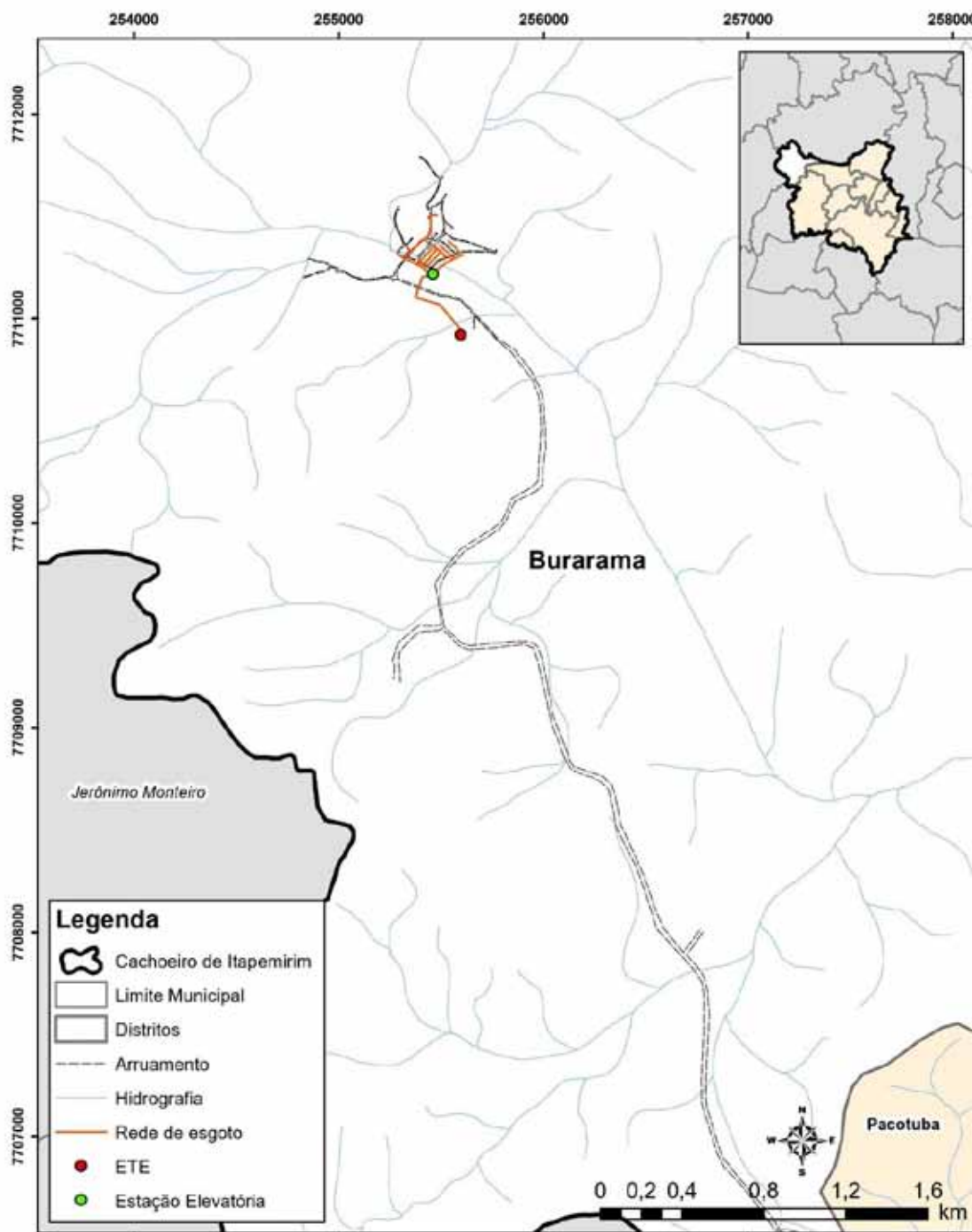
Figura D-197 – Sistema de esgotamento sanitário do distrito de Burarama.
