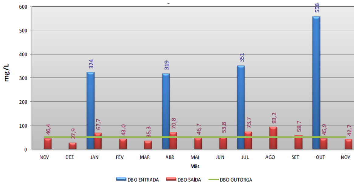
Figura AC-179 - Resultados de DBO na ETE Córrego dos Monos.
