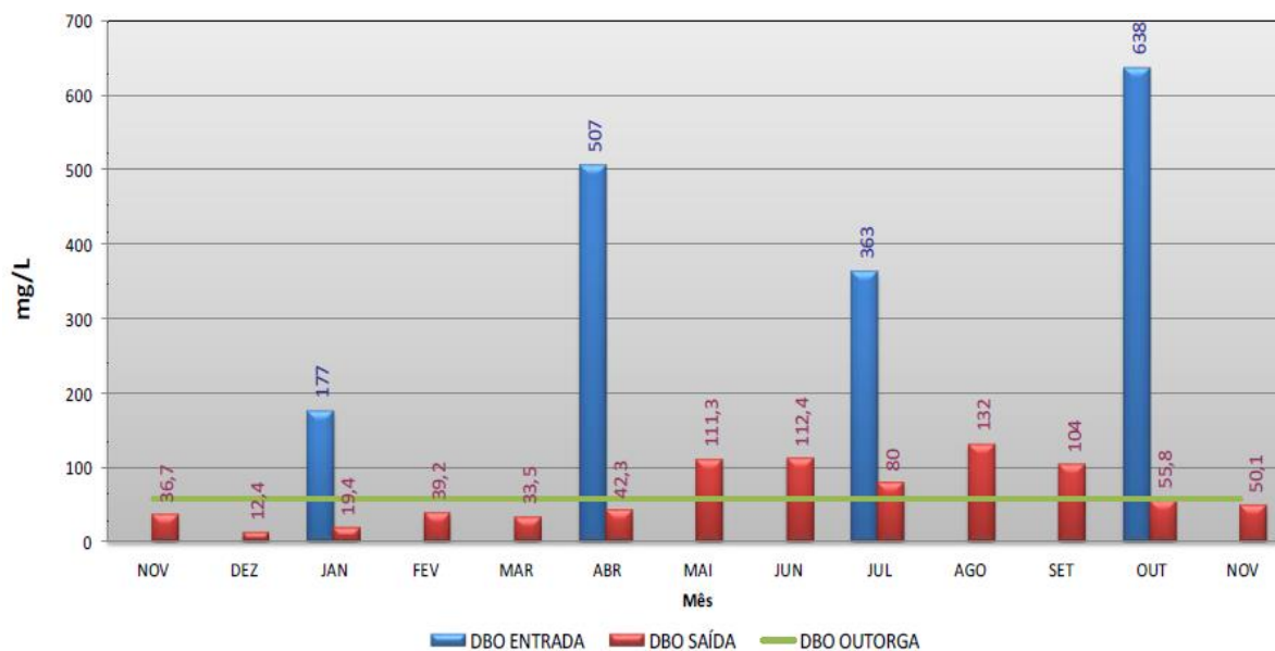
Figura AC-178 - Resultados de DBO na ETE Conduru.
