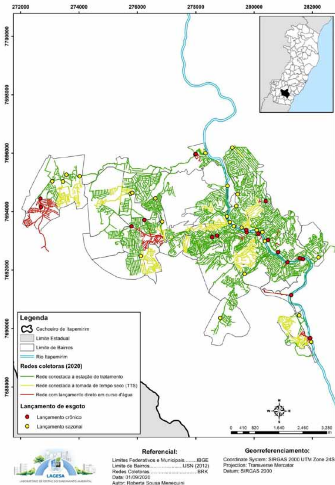
Figura 10-130 – Diagnóstico Atual (2020) das redes coletoras de esgoto presente no município.
