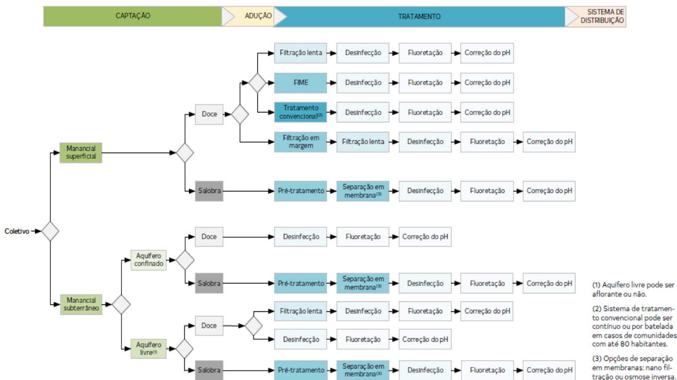
Figura O-283 - Matriz tecnológica de soluções coletivas para o abastecimento de água, segundo FUNASA.
