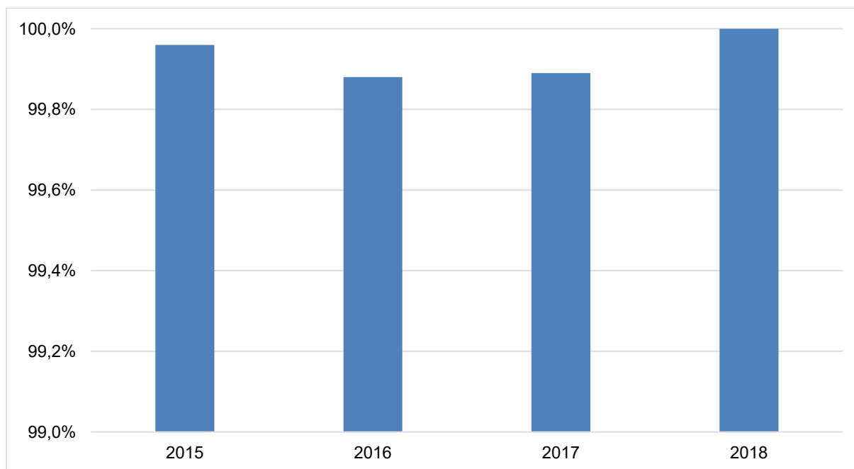
Figura 9-87 – Índice de hidrometração do sistema de abastecimento de água no município de Cachoeiro de Itapemirim (2015-2018).
