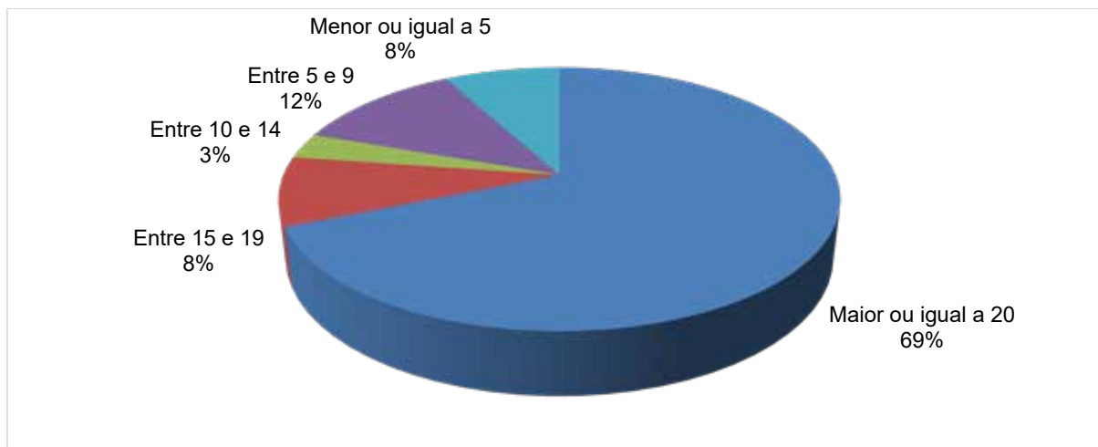
Figura 9-41 - Percentual da idade média (anos) das redes de abastecimento de água.
