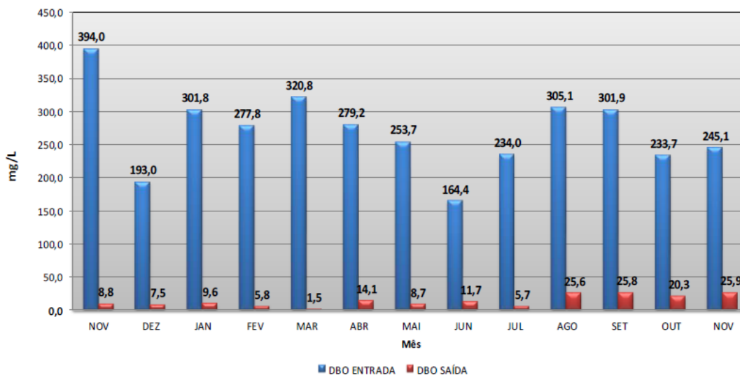
Figura AC-173 – Resultados de DBO na ETE Coronel Borges.
