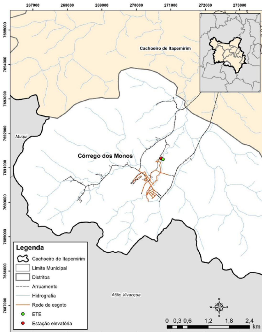
Figura D-199 - Sistema de esgotamento sanitário do distrito Córrego dos Monos.
