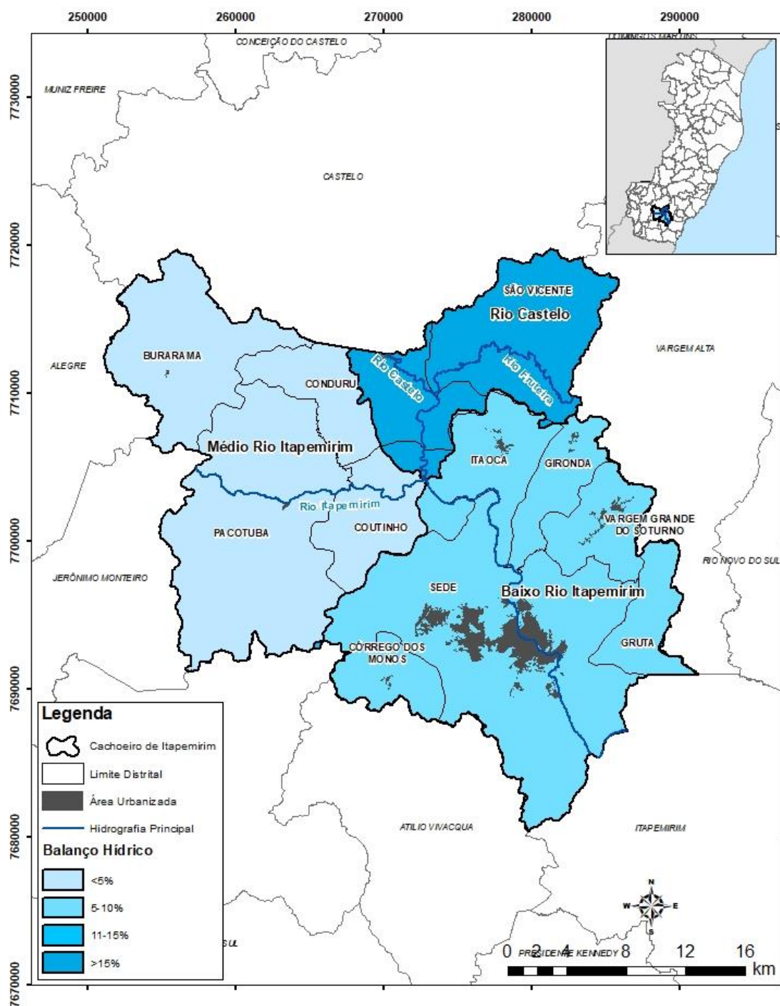
Figura 9-99 - Balanço hídrico em razão da Q90 na Bacia Hidrográfica do Rio Itapemirim, por Unidade de Planejamento do Plano de Bacias em Cachoeiro de Itapemirim.
