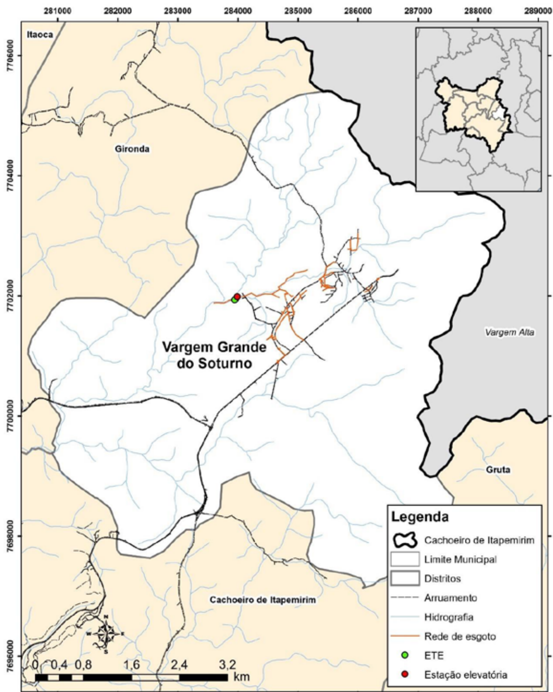
Figura D-205 - Sistema de esgotamento sanitário do distrito Vargem Grande do Soturno.
