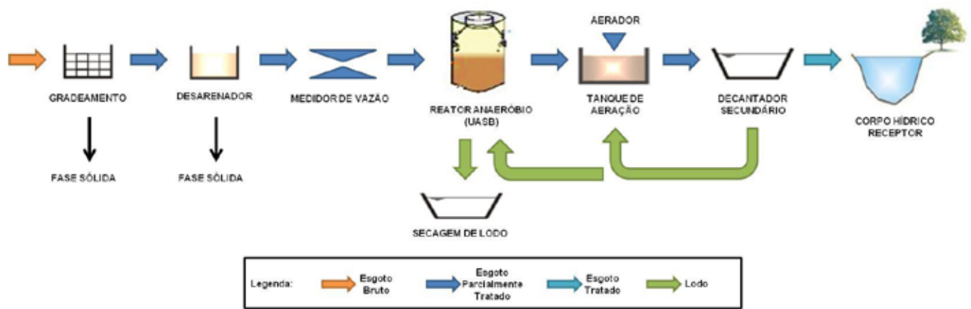
Figura 16-164 - Etapas de tratamento de esgotos pelo sistema de reator UASB + lodos ativados.
