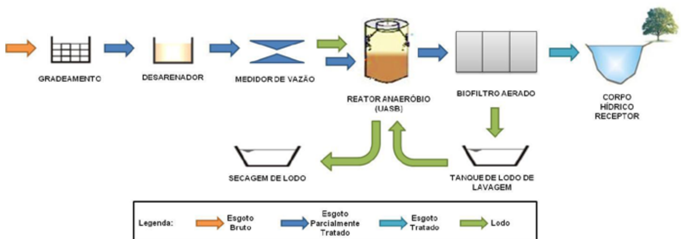
Figura 16-162 - Etapas de tratamento de esgotos pelo sistema UASB + biofiltro aerado submerso.
