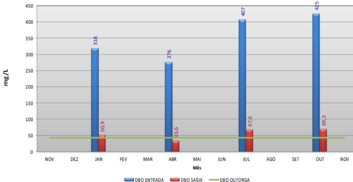
Figura AC-182 - Resultados de DBO da ETE Itaoca.
