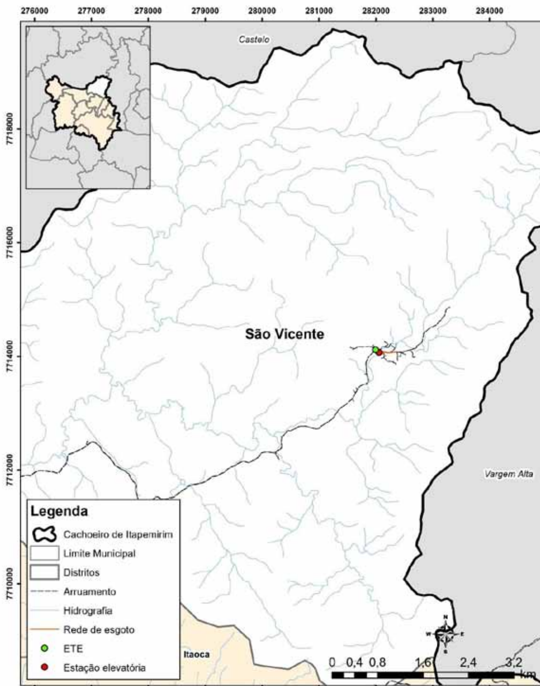
Figura D-204 - Sistema de esgotamento sanitário do distrito São Vicente.
