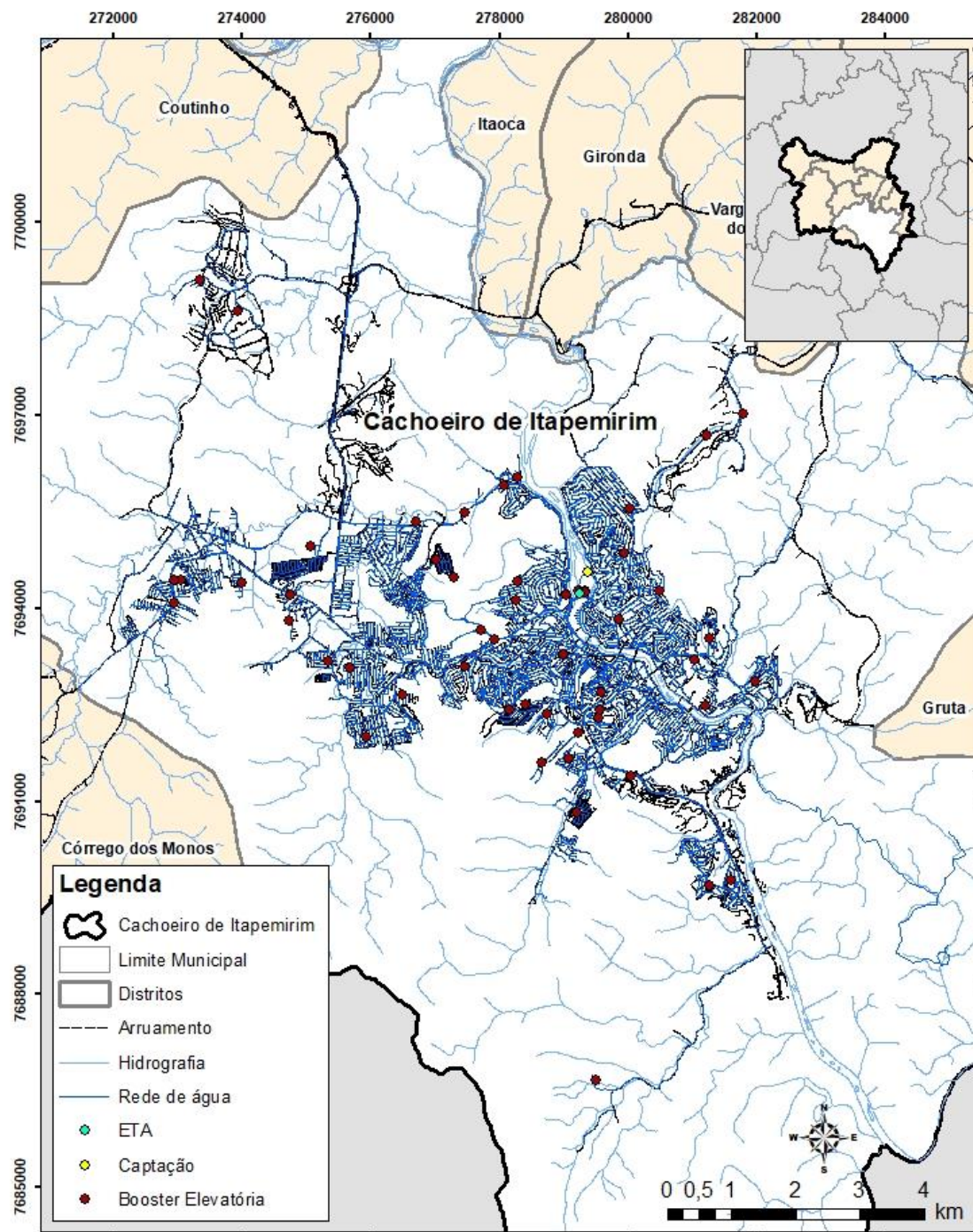
Figura C-195 - Sistema de abastecimento de água da Sede Municipal.
