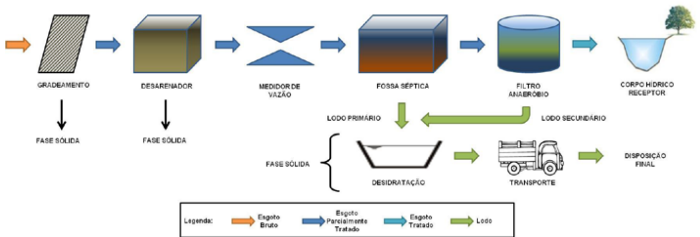
Figura 16-165 - Etapas de tratamento de esgotos pelo sistema de fossa séptica e filtro anaeróbio.
