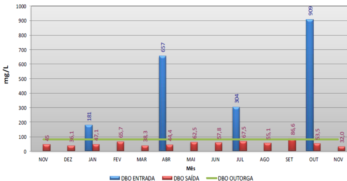
Figura AC-181 - Resultados de DBO da ETE Gironda.
