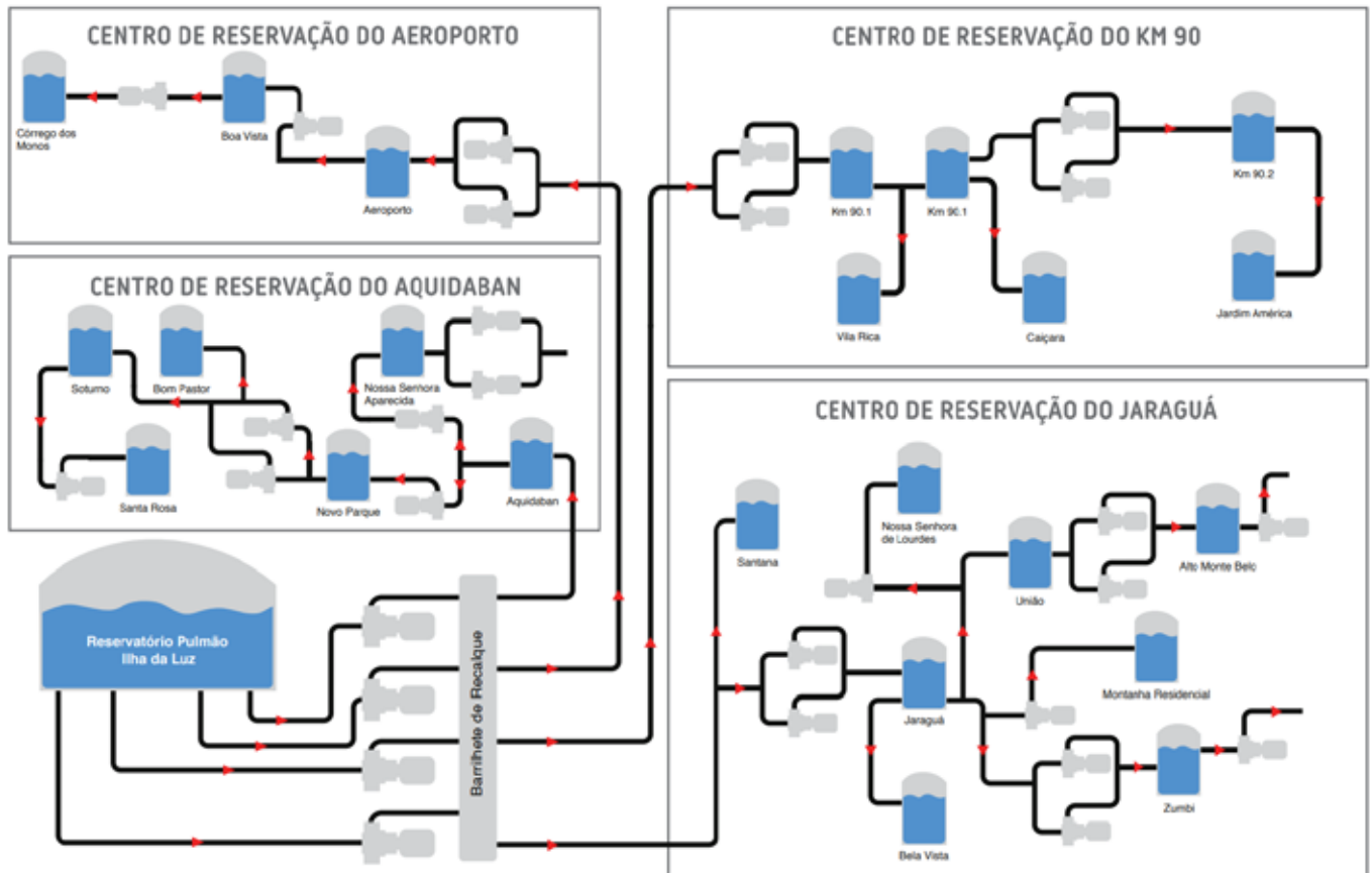
Figura 9-44 - Sistemas de reservação e distribuição de água da sede de Cachoeiro de Itapemirim.
